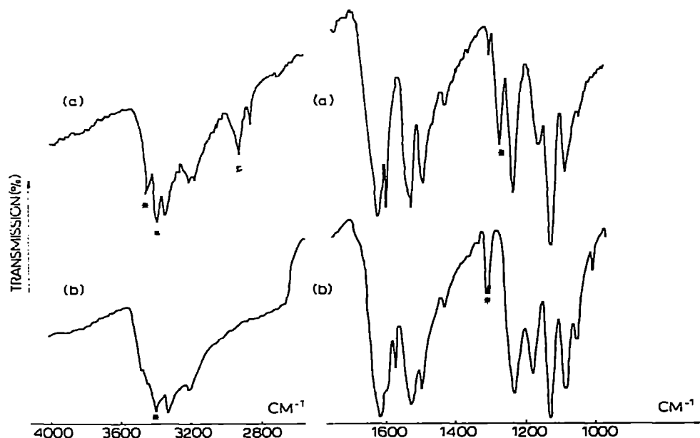
Fig. 2. Spectres IR de la sulfaguanidine. (a) Initiale; (b) comprimée à 450 MPa.
