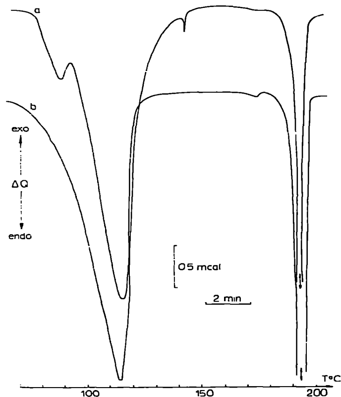
Fig. 5. Courbes d'analyse calorimétrique différentielle de la sulfaguanidine monohydratée. (a) Initiale; (b) comprimée à 450 MPa. Conditions opératoires: prise d'essai 6,0 mg; capsules ordinaires non serties; vitesse de chauffage 10°C min -1 .
