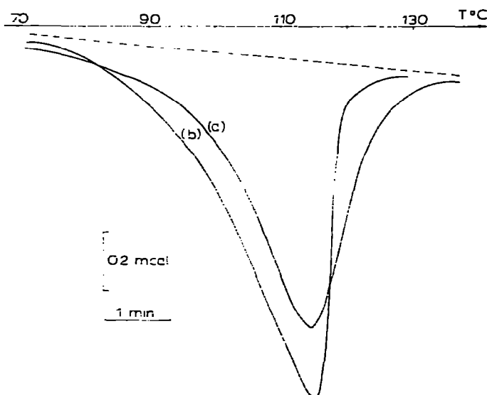
Fig. 7. Courbes d'analyse calorimétrique différentielle de la sulfaguanidine monohydratée. (a) Initiale; (b) comprimée à 450 MPa. Conditions opératoires: prises d'essai 2,10 mg; capsules serties; vitesse de chauffage 10^{\circ}\text{C min}^{-1} ; sensibilité 0,2 \text{ mcal sec}^{-1} \text{ pouce}^{-1} ; base de temps 1 \text{ min pouce}^{-1} .
