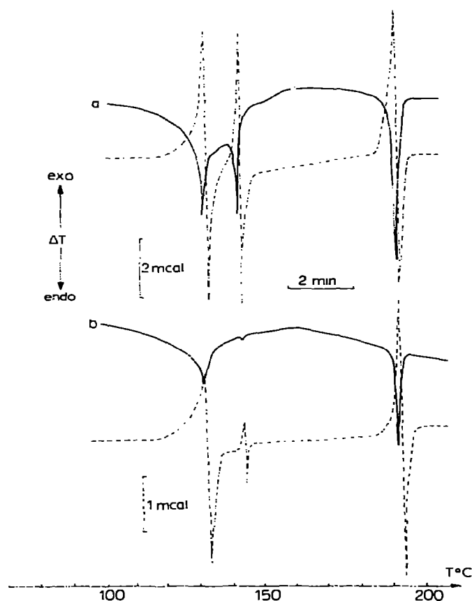
Fig. 4. Courbes d'analyse thermique différentielle de la sulfaguanidine monohydratée. (a) Initiale; (b) comprimée à 450 MPa. (—) Courbe ATD; (- - - -) courbe dérivée. Conditions opératoires: prise d'essai 6 mg environ; vitesse de chauffage 10 ^{\circ}\text{C min}^{-1} .
