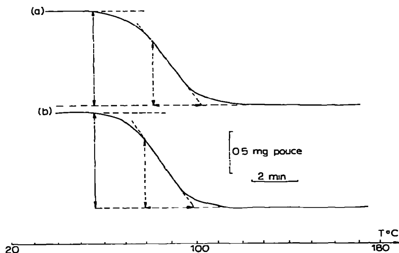
Fig. 3. Courbes thermogravimétriques de la sulfaguanidine monohydratée. (a) Initiale; (b) comprimée à 450 MPa. Conditions opératoires: prise d'essai 14,4 mg; vitesse de chauffage 10°C min -1 .
