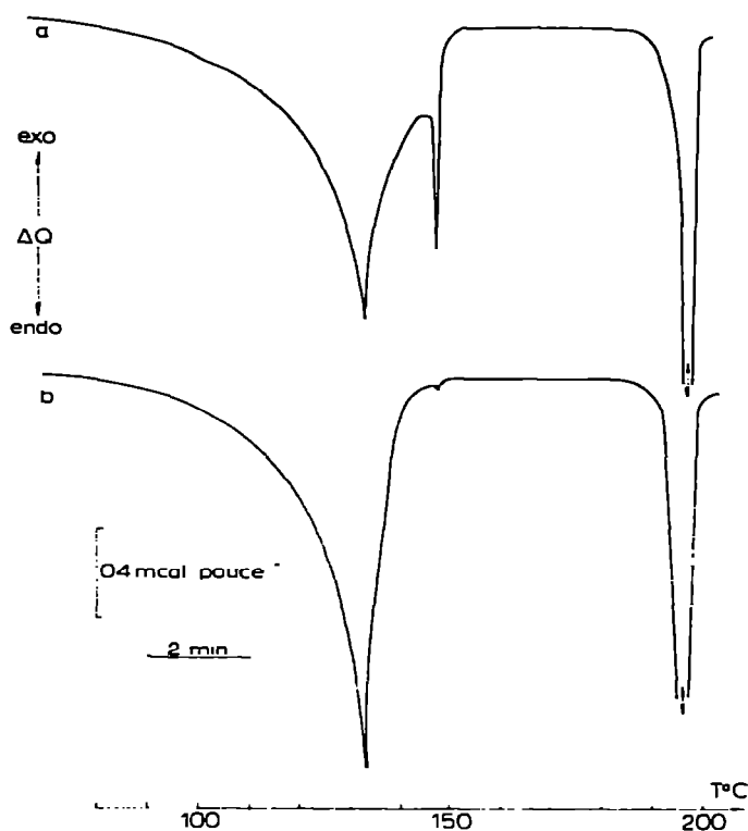
Fig. 6. Courbes d'analyse calorimétrique différentielle de la sulfaguanidine monohydratée. (a) Initiale; (b) comprimée à 450 MPa. Conditions opératoires: prises d'essai 4,2 mg; capsules serties; vitesse de chauffage 10^{\circ}\text{C min}^{-1} .
